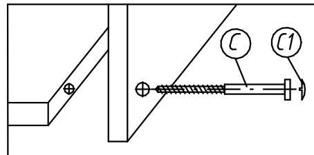
Крепление винта саморезного (комплект №19)
